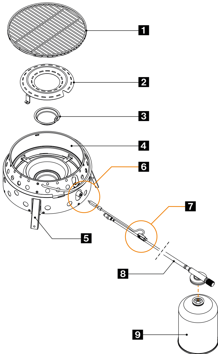
Σχ.: Συναρμολόγηση ψησταριάς αερίου Atago
