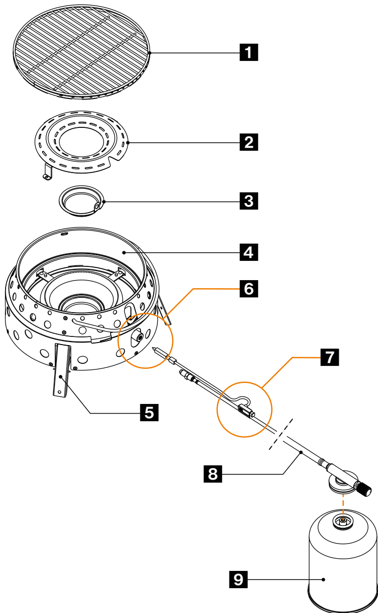
Attēls: Atago gāzes grila montāža
