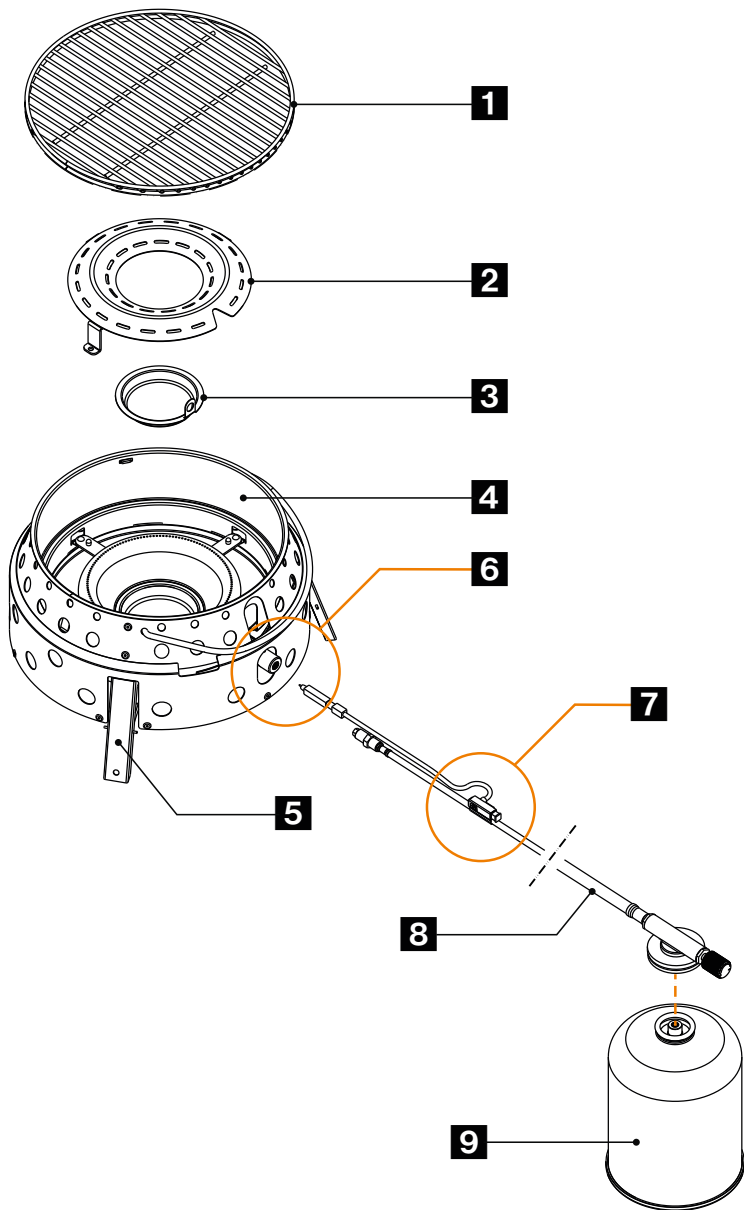
Фигура: Сглобяване на газово барбекю Atago
