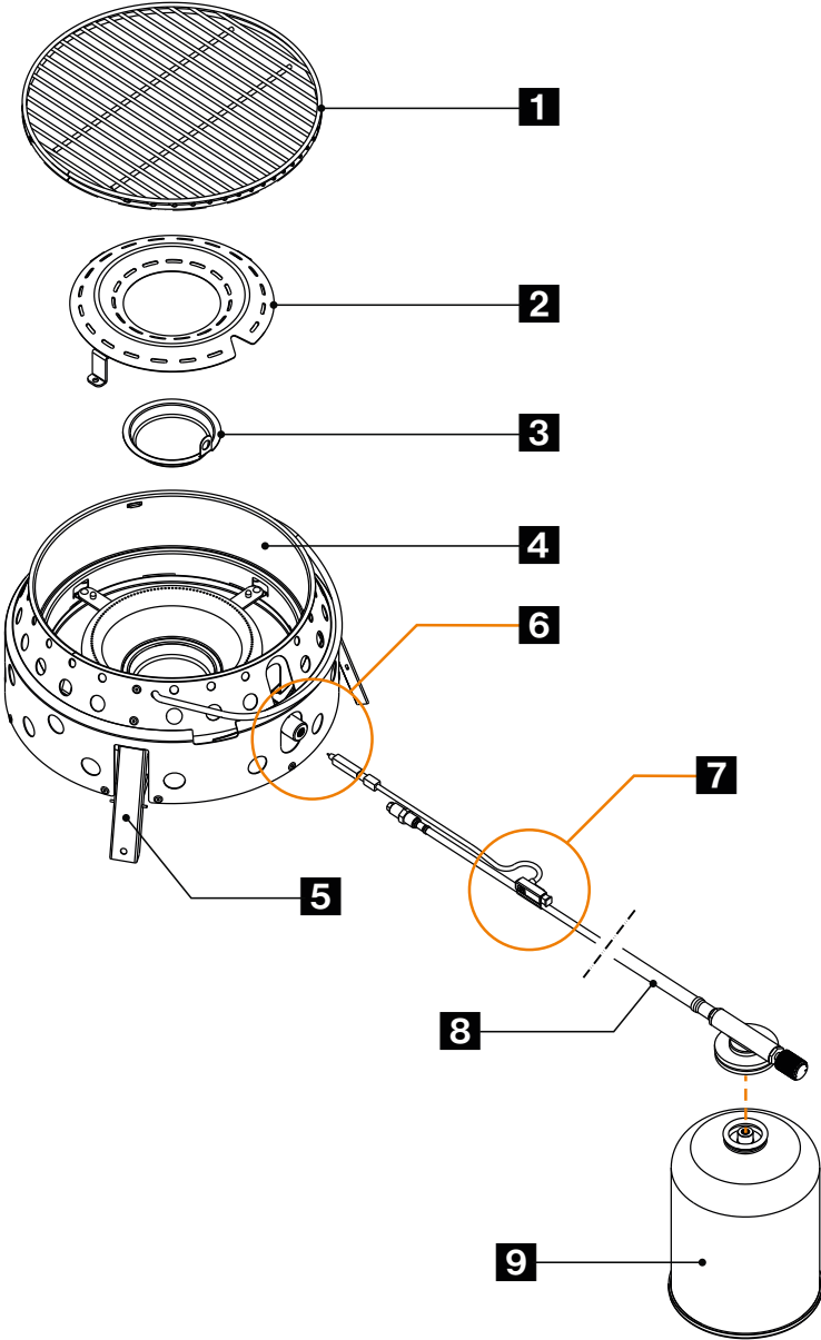
Şekil: Atago gazlı barbekü düzeneği
