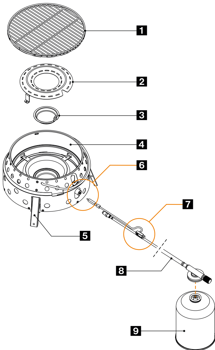
Ábra: Atago gázgrill összeszerelése
