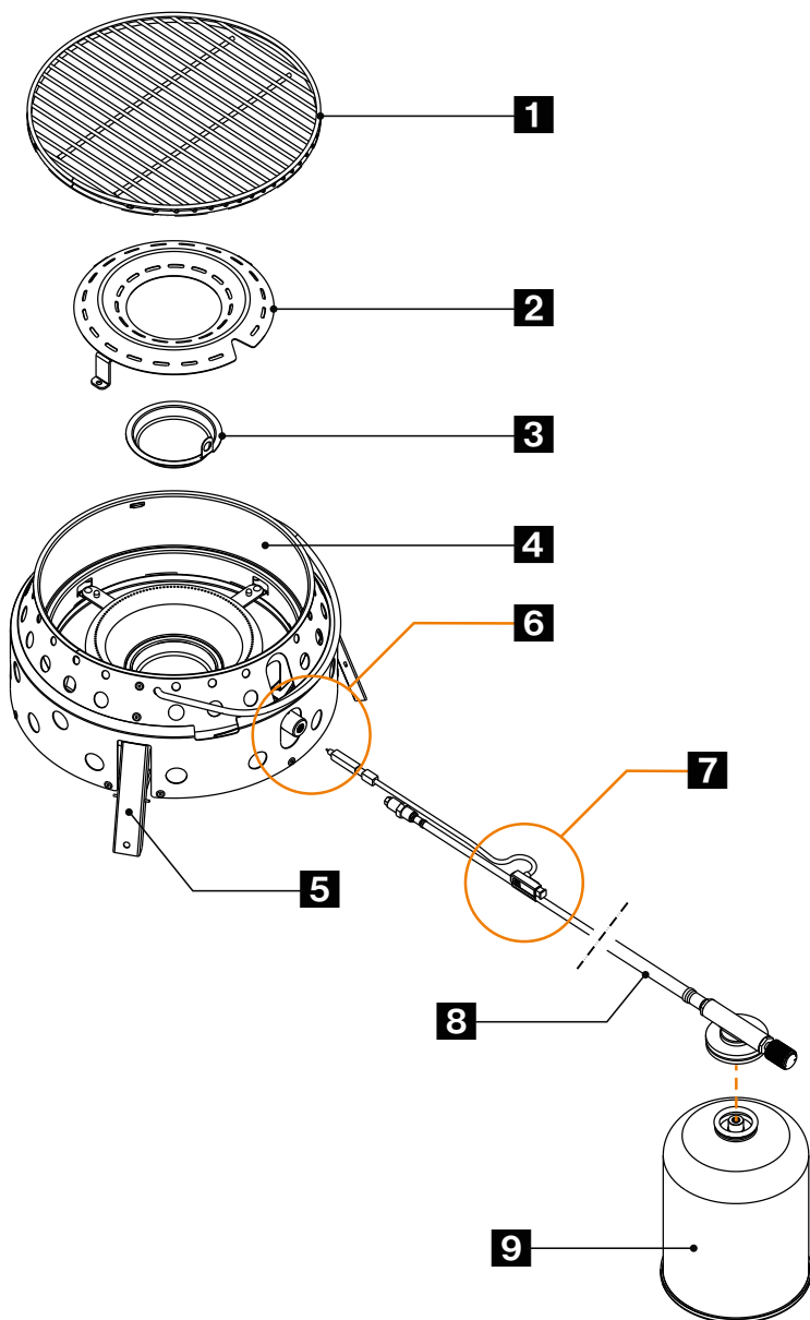
Fig.: Montering av gasogrill Atago
