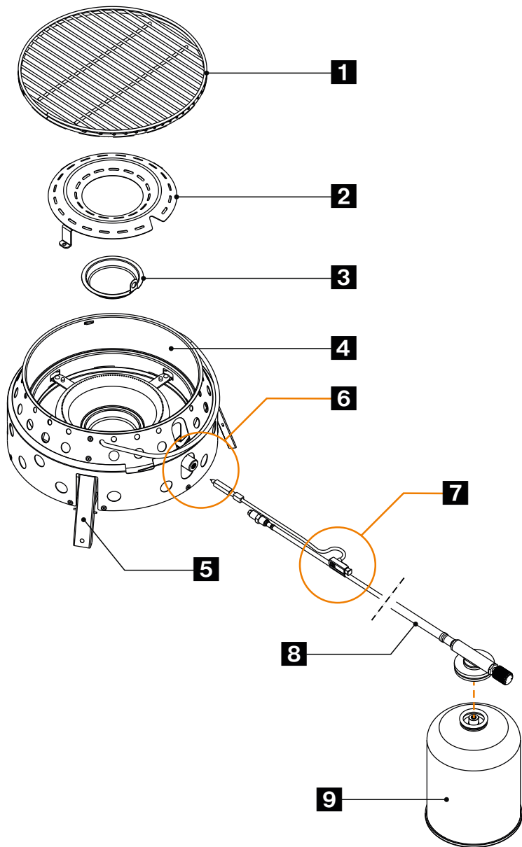
Obr.: Sestava plynového grilu Atago
