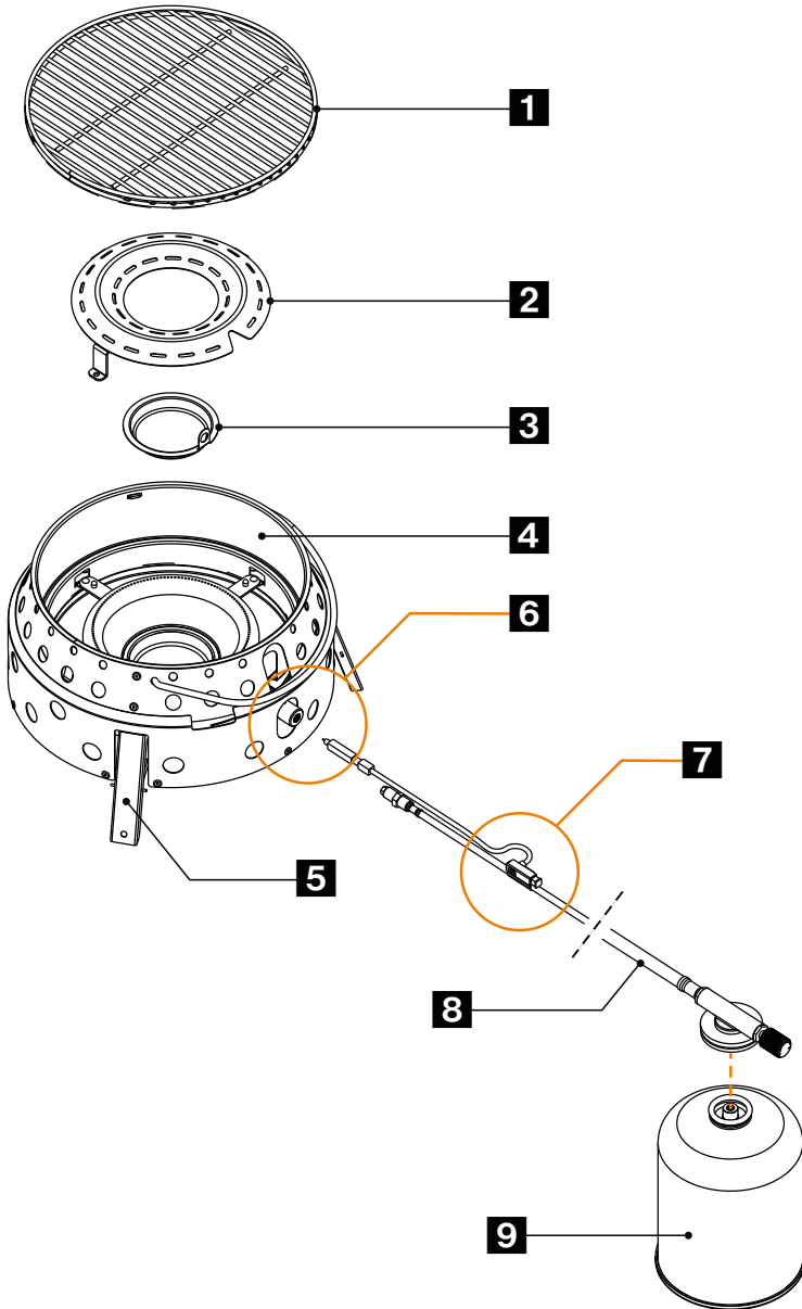
Afb.: Atago gasbarbecue montage
