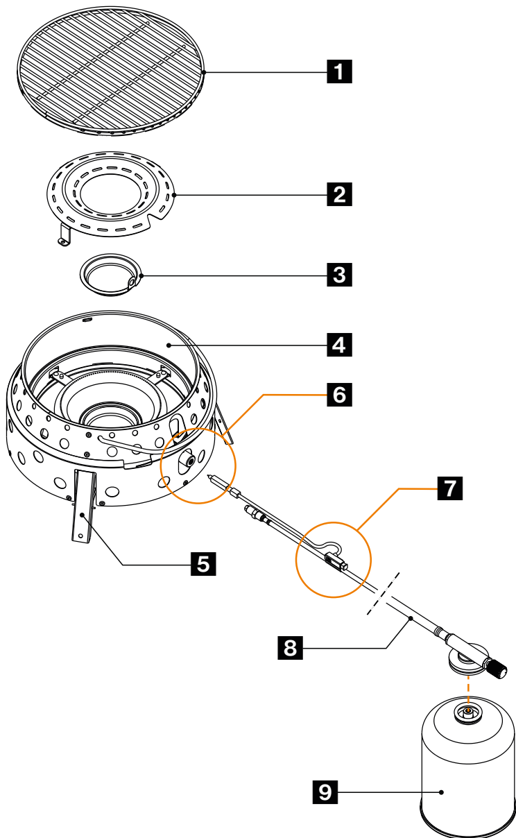
Fig.: Montagem da churrasqueira a gás Atago
