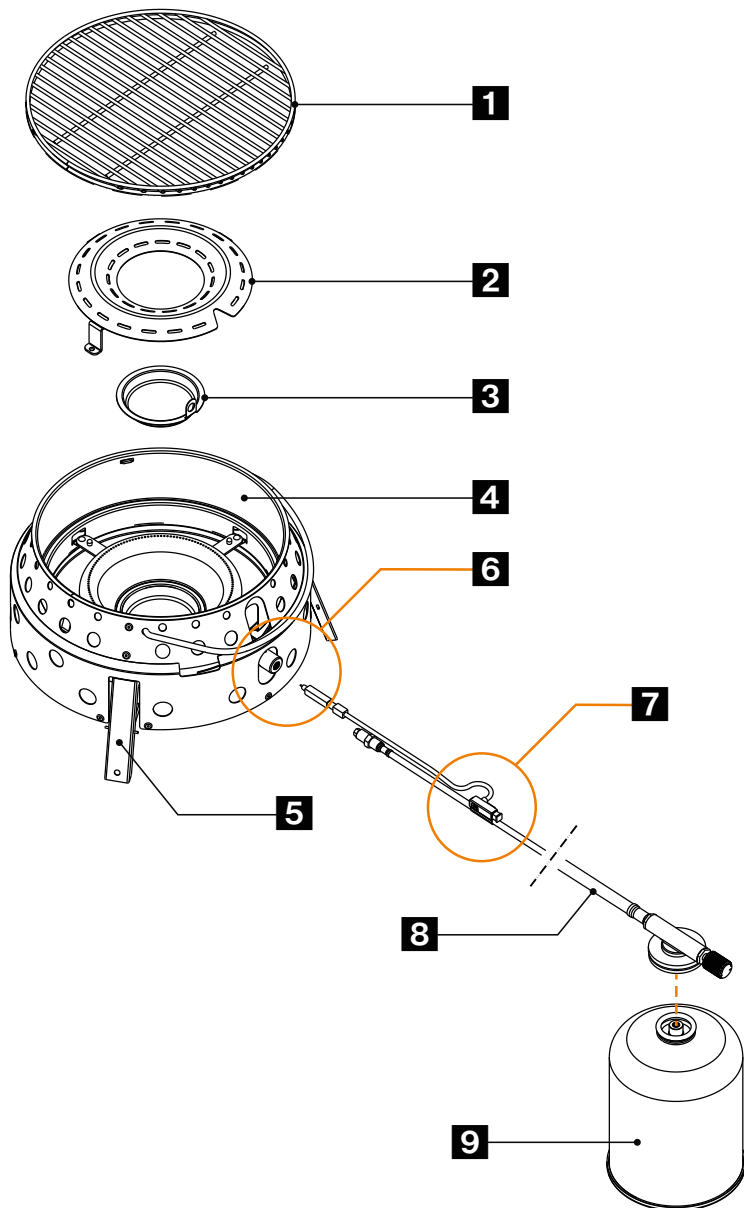
Rys.: Montaż grilla gazowego Atago
