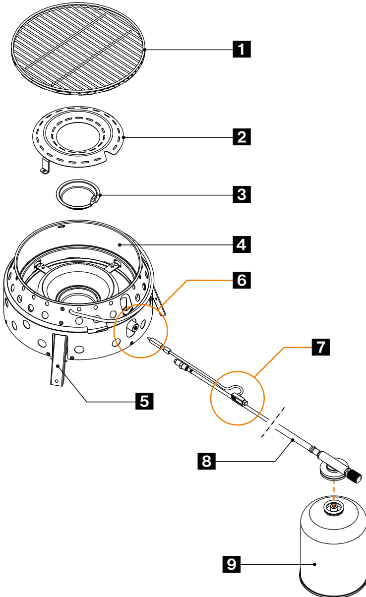
Fig. : Montage du barbecue à gaz Atago
