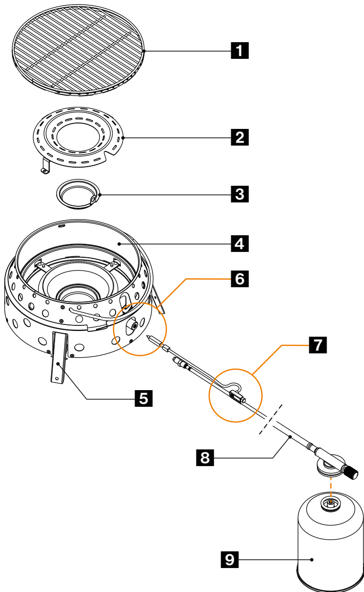
Pav.: „Atago“ dujinės kepsninės surinkimas
